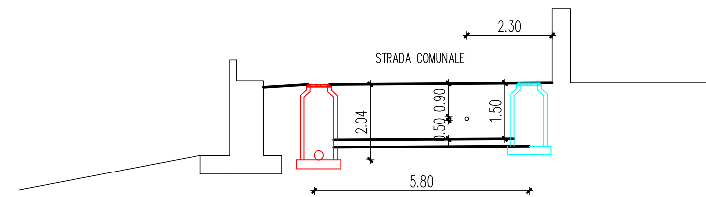
SEZIONE TIPO SCALA 1/100
