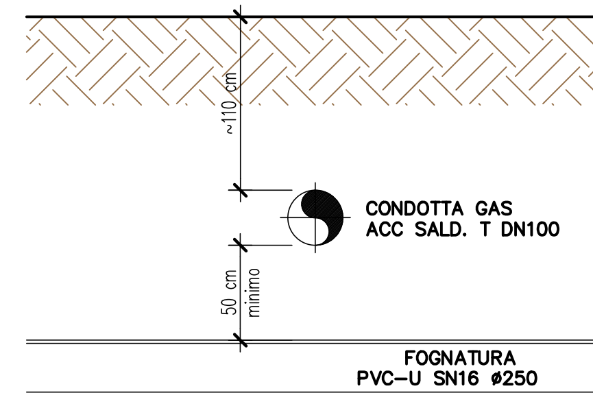
ATTRAVERSAMENTO DI CONDOTTA GAS
